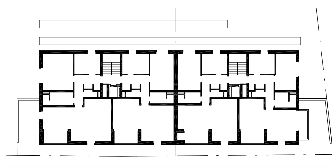
Plan du 1er étage
