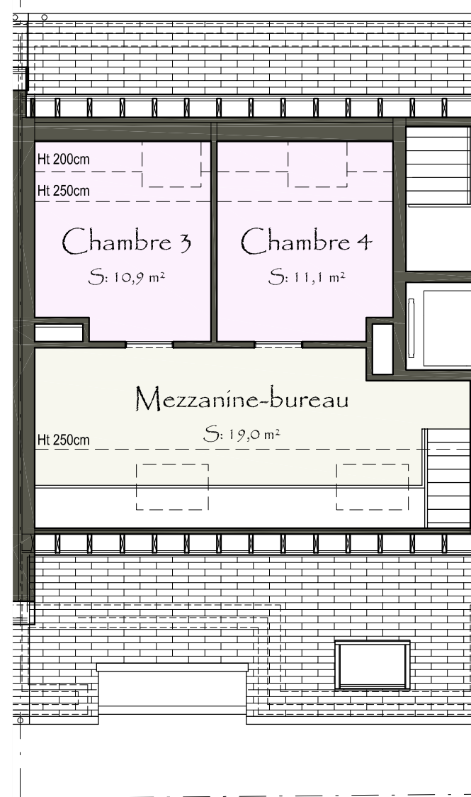
Plan du 2ème étage
