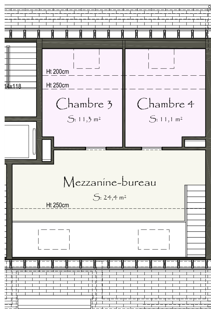
Plan du 2ème étage
