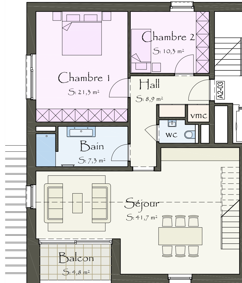
Plan du 1er étage
