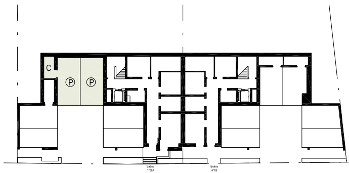
Plan du rez de chaussée
