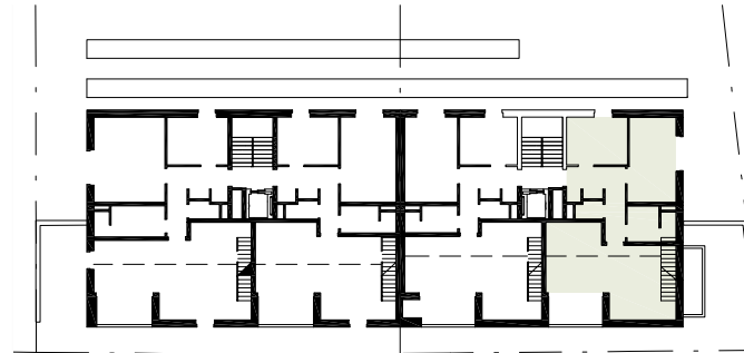
Plan du 2ème étage
